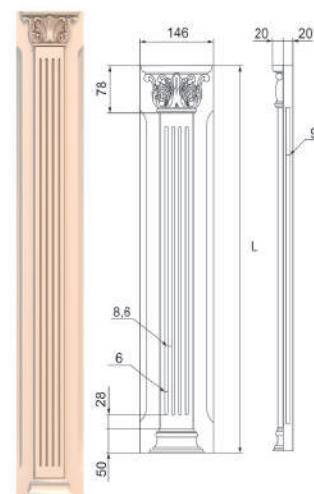
Пилястра 1
