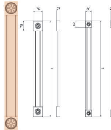
Колонна 8
