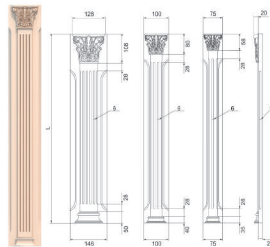
Пилястра 2
