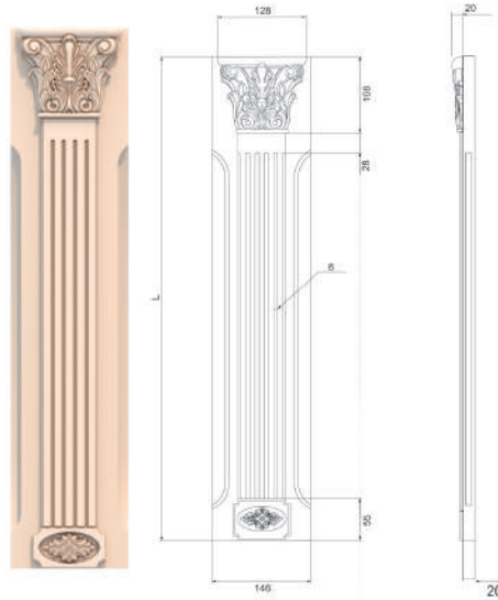
Пилястра 4
