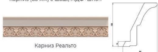
Карниз (83 мм) с шаш., МДФ+шпон
