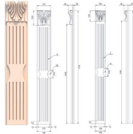
Пилястра 10
