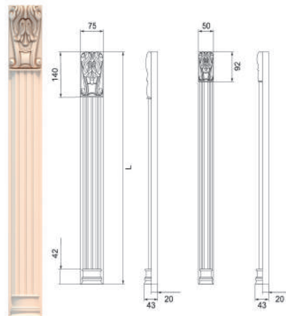
Колонна 7
