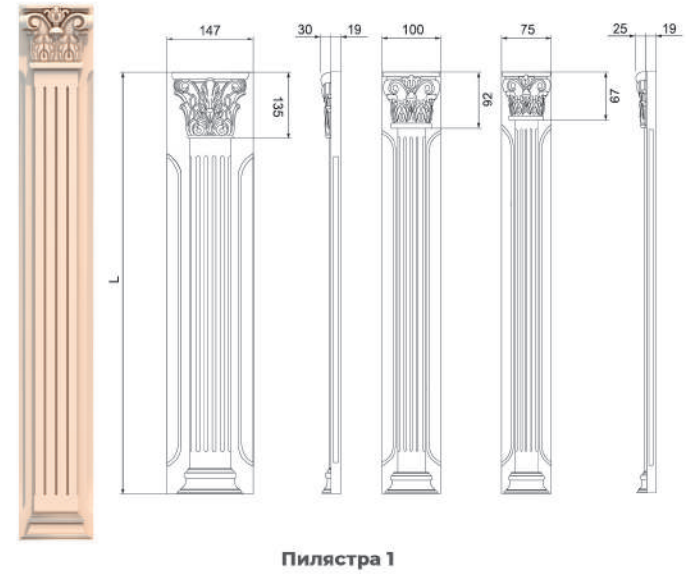
Пилыстра 1
