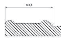
Сечение профиля с плоской филёнкой
