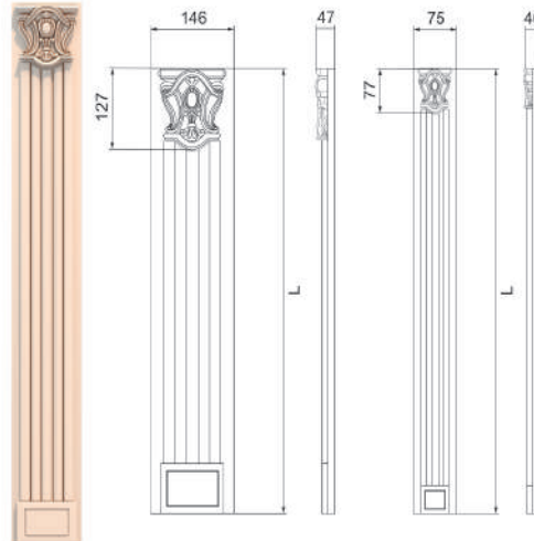
Пилястра 8
