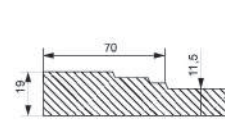
Сечение профиля
