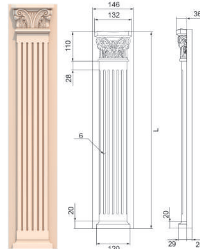
Пилястра 5
