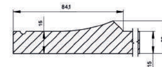
Сечение профиля
