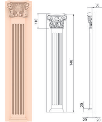
Пилястра 6
