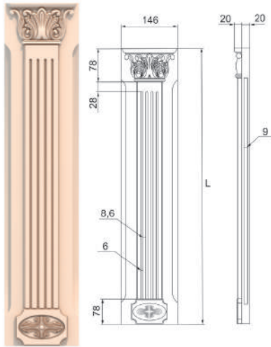
Пилястра 3
