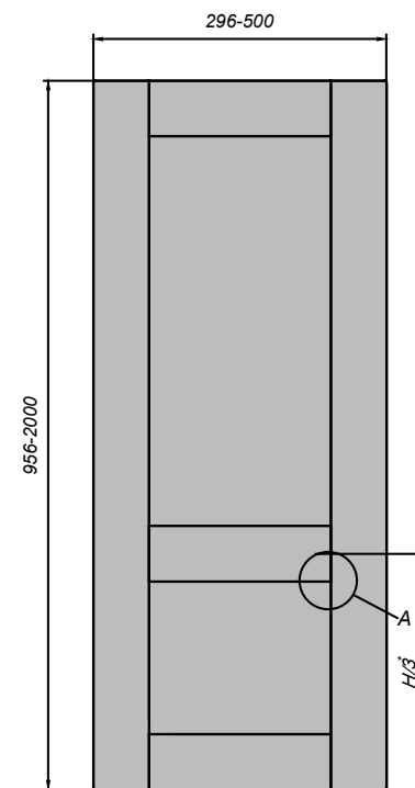
Глухой фасад с 1-м импостом (вставка 3 мм)
