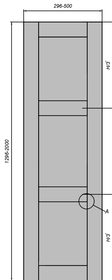
Глухой фасад с 2-мя импостами (вставка 3 мм)
