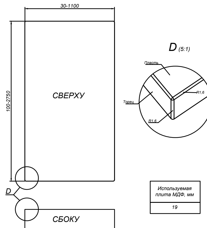
ПАНЕЛЬ БЕЗ ТОРЦА
