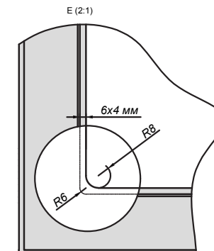
Выборка на обратной стороне
