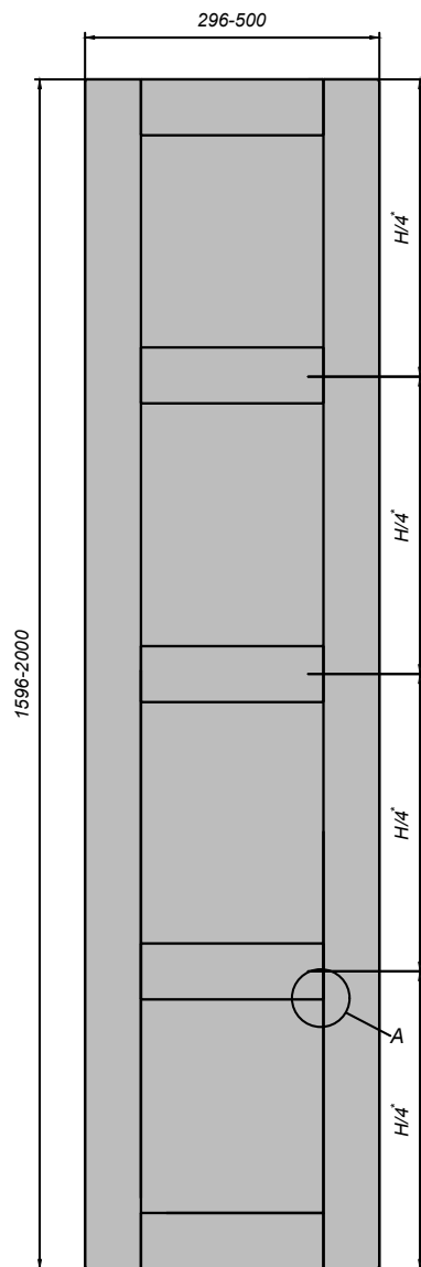
Глухой фасад с 3-мя импостами (вставка 3 мм)
