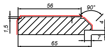
B-B (5:1)
