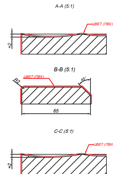
E (2:1)
