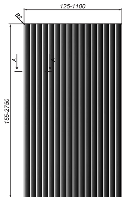
Глухой фасад
