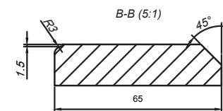
Профиль фасадов витринного типа
