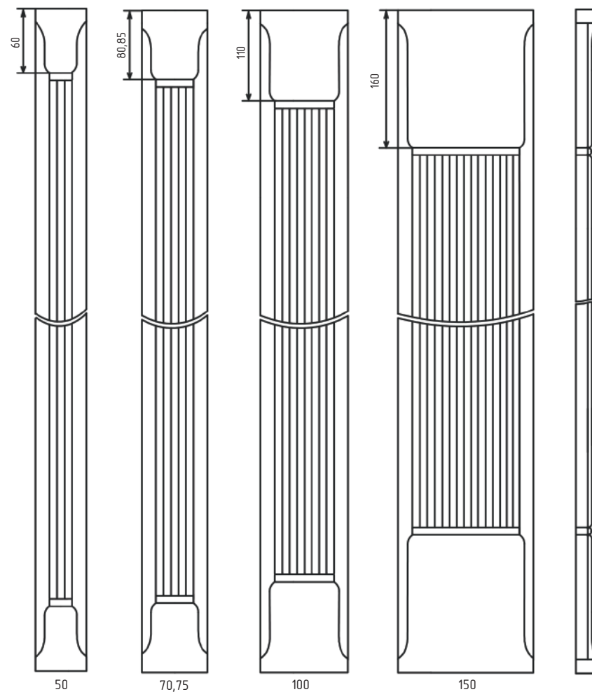
Пилястра №3
