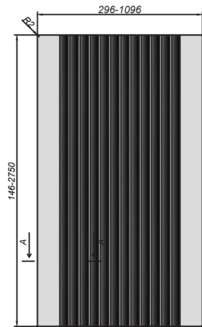
Глухой фасад
