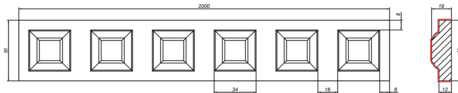
СВЕТОВАЯ ПЛАНКА 2
