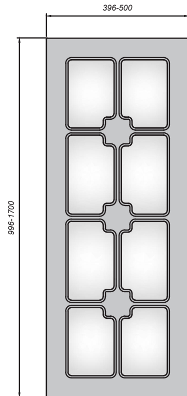
Витрина 2 со стеклом 8 окон*
