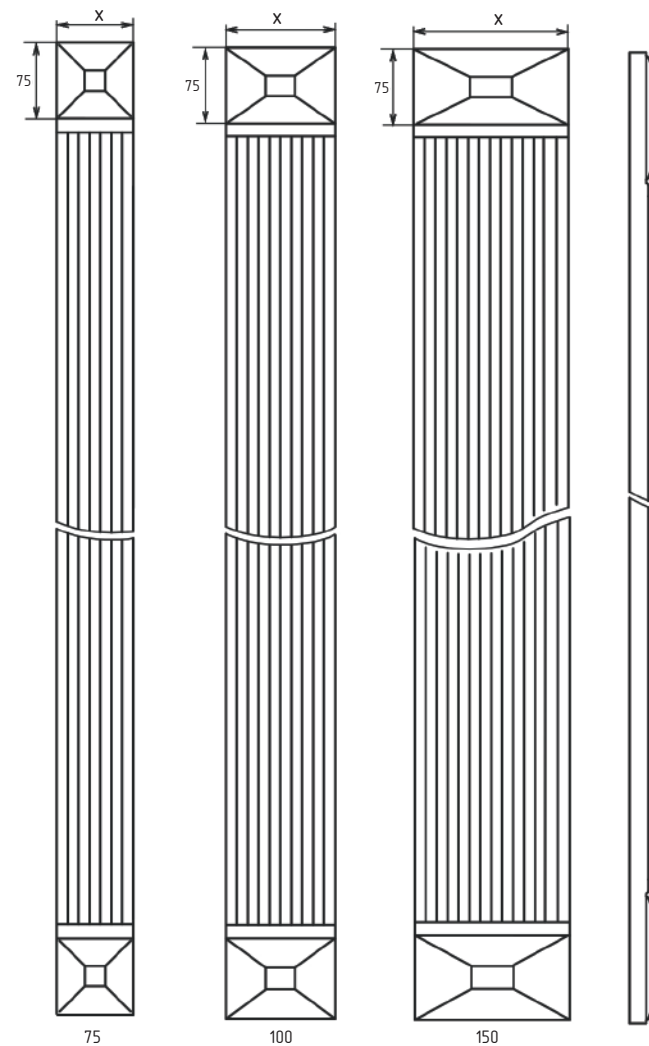
Пилястра №6
