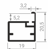
MZ 07 Профиль фасадный
