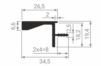
KB 93 Профиль врезной для верхних баз
