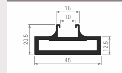
TS 101 new Профиль вертикальный
