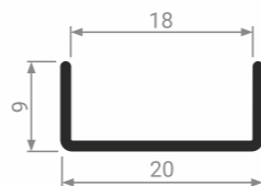
C18-02 Профиль фасадный
