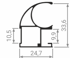
MS 125V Профиль вертикальный асимметричный Облегченная версия MS 125
