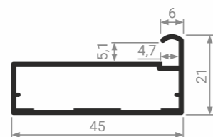
MZ 09 Профиль фасадный
