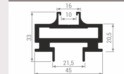
TS 102 new Профиль горизонтальный
