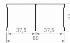
MS 310C Направляющая верхняя
