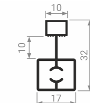
MS 413 Профиль разделительный
