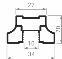
MS 160 Профиль вертикальный
