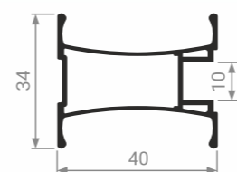
MS 155 Профиль вертикальный
