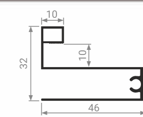
MS 223 Профиль горизонтальный нижний
