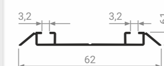
MS 320C Направляющая нижняя
