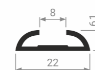
MS 341 Направляющая для распашной двери
