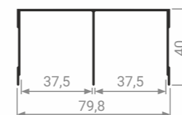
MS 310 Направляющая верхняя
