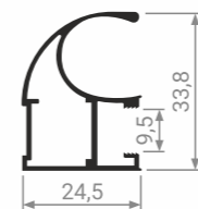
MS 125C Профиль вертикальный асимметричный Облегченная версия MS 125
