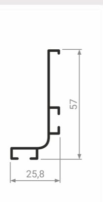
Уголок внешний для профиля L-образного 90°
