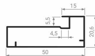
MZ 04 Профиль фасадный
