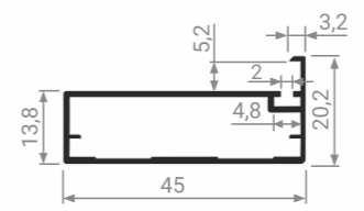
MZ 17 Профиль фасадный
