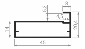
MZ 13 Профиль фасадный
