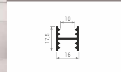
TS 105 Профиль разделительный
