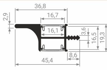
KB 94 Профиль врезной с двухсторонней подсветкой
