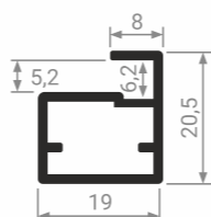
MZ 02 Профиль фасадный
