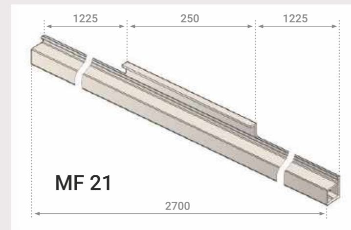
MF 21 Профиль - ручка
