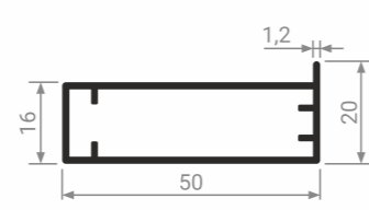
MZ 10 Профиль фасадный
