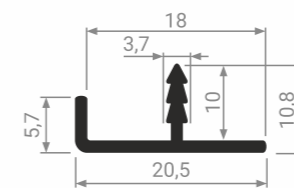
T 18-03 Профиль врезной
