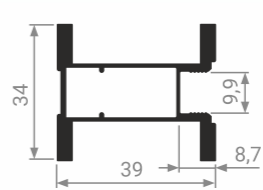
MS 170 Профиль вертикальный
