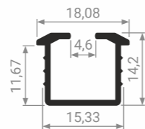
MS 30 Верхняя/нижняя направляющая
