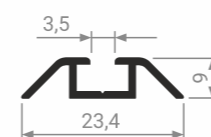
MS 340 Направляющая одинарная нижняя
