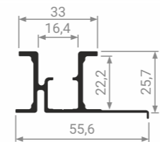
MT 902 V Верхняя направляющая
