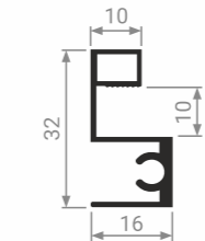
MS 213 Профиль горизонтальный верхний
