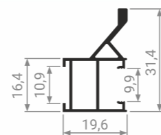
MS 145 Профиль вертикальный
