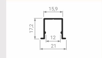
MS 185 Профиль врезной нижний для деревянных дверей
