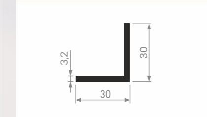
Уголок для крепления направляющей к стене
