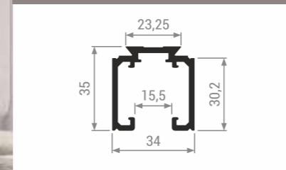
TS 103 Направляющая для телескопической системы
