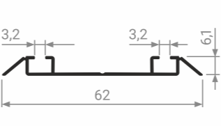
MS 320C Направляющая нижняя
