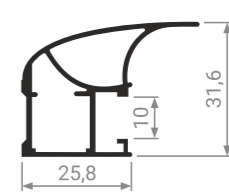
MS 130 Профиль вертикальный асимметричный
