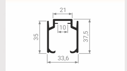
MS 184 Направляющая для подвесной системы
