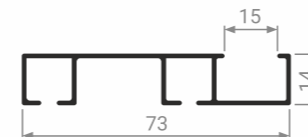
MS 52 Направляющая верхняя
