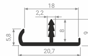
T 18-02 Профиль врезной
