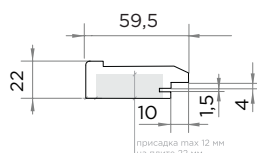
Паз под уплотнитель
