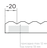
А-А
