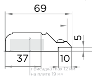
Б-Б
