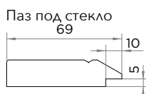
Б-Б
