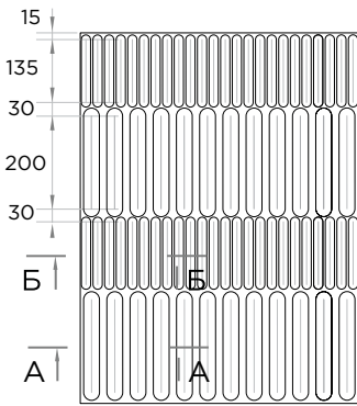
Глухой 1
