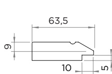
Паз под стекло
