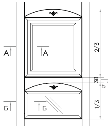
Составной
