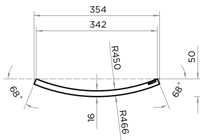
R 450/16 выпуклый
