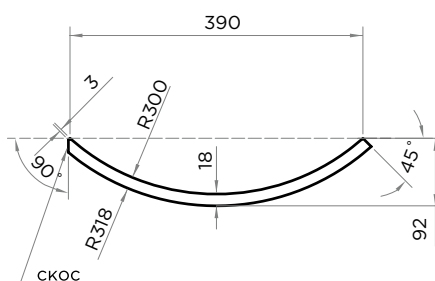
R 300/18 вогнутый
