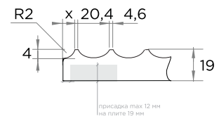
Б-Б
