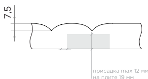
A-A
