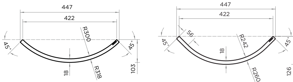
R 300/18 выпуклый
