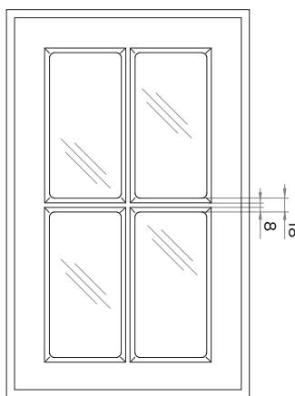
Переплёт
