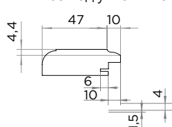
Паз под уплотнитель
