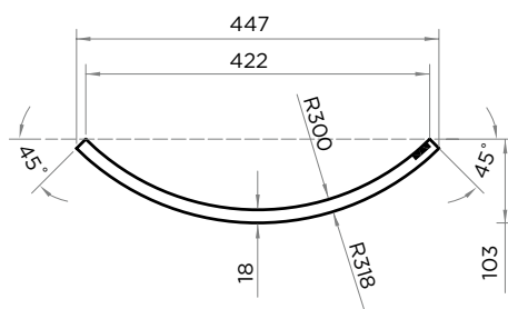
R 300/18 выпуклый
