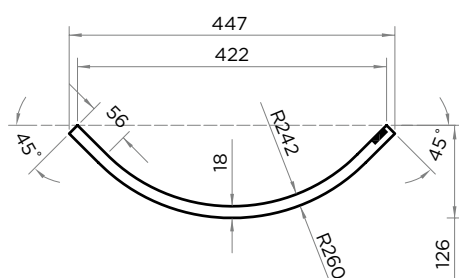
R 242/18 выпуклый
