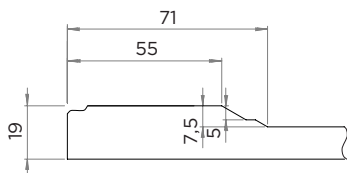
Ящик "Браво"
