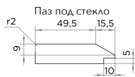
Б-Б
