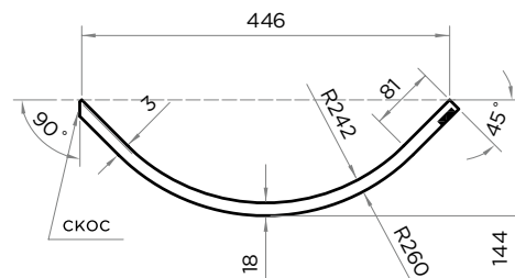
R 242/18 вогнутый
