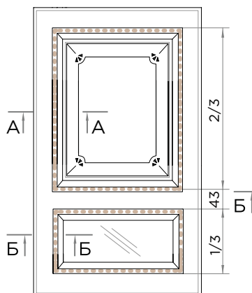
Ящик 2
