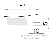
Паз под стекло
