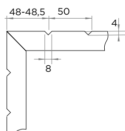
В-В
