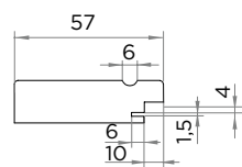
Паз под уплотнитель (19, 22 мм)
