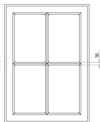
Тонкий Переплет
