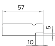
Б-Б Паз под стекло
