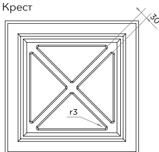
Крест
