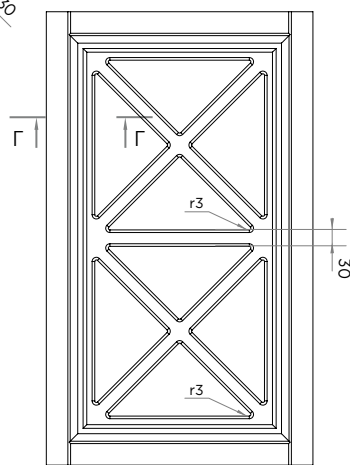
Двойной крест
