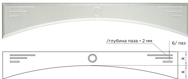
Арка А1
