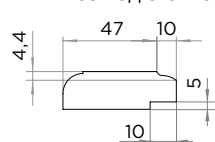
Паз под стекло
