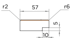
Б-Б Паз под стекло
