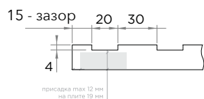
Расположение на гарнитуре
