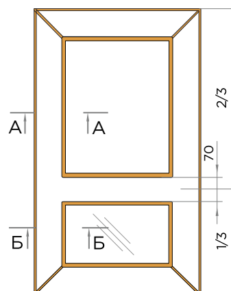
Составной
