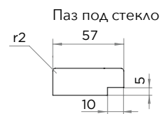
В-В
