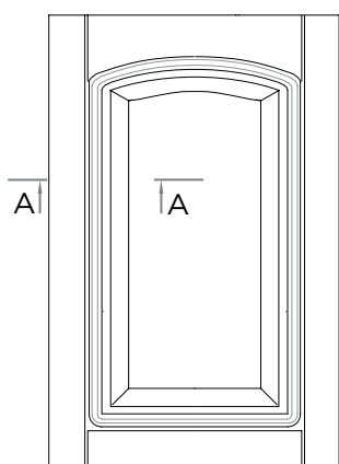
Глухой фасад
