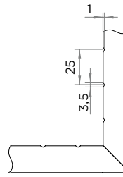
В-В
