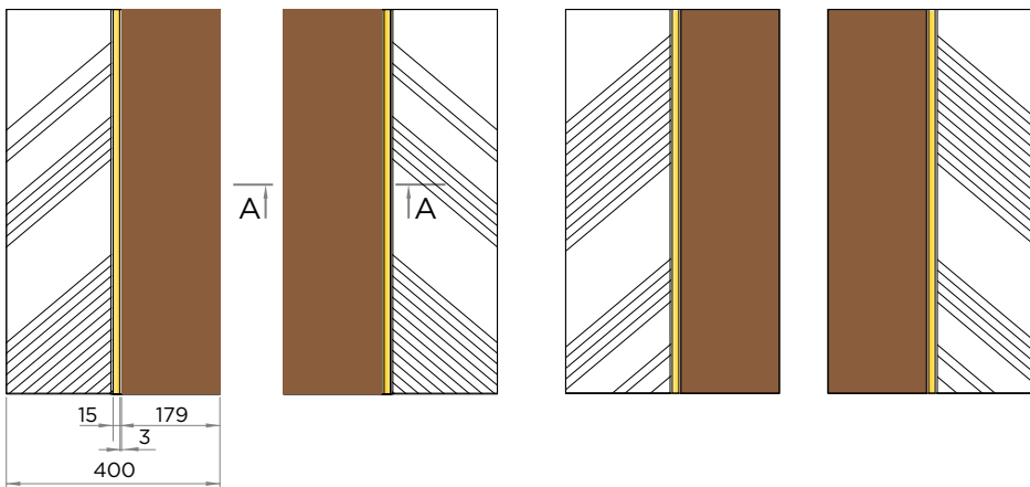
Глухой фасад 1
