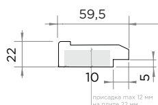
Б-Б Паз под стекло
