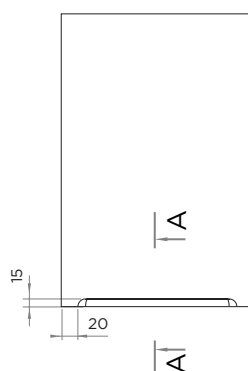
Глухой фасад 1 (верхняя база)
