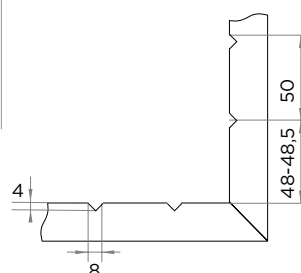
Г-Г
