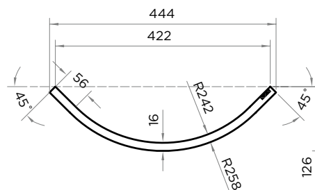
R 242/16 выпуклый
