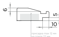
Б-Б Паз под стекло
