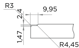
Торец Тип 6
