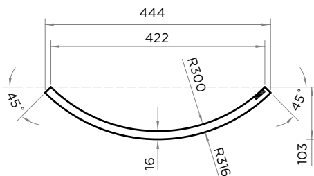
R 300/16 выпуклый
