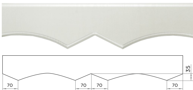
Арка А4
