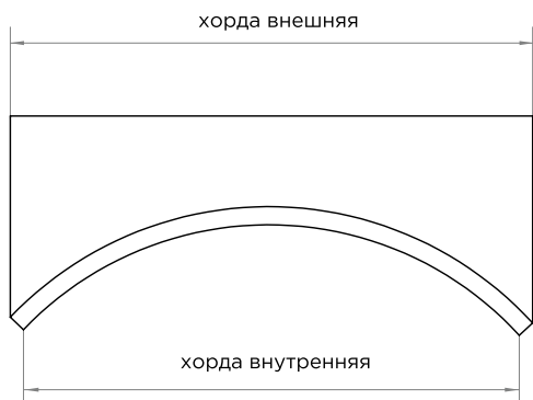
Выпуклый фасад
