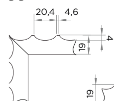
Б-Б
