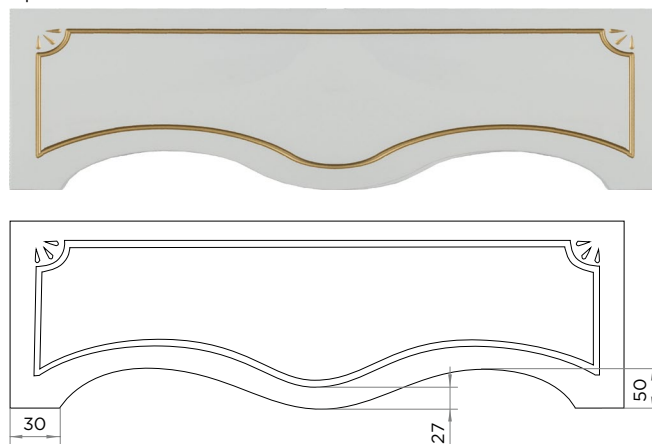
Арка А6
