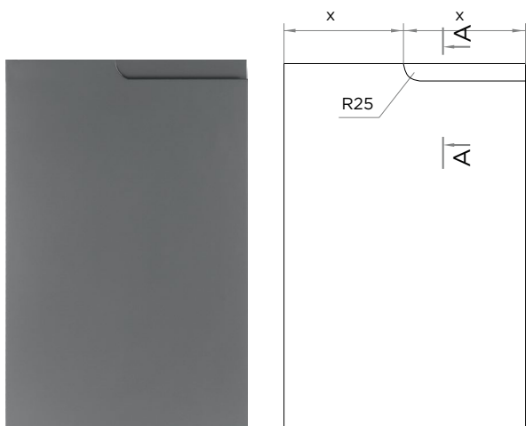
Глухой фасад 2
