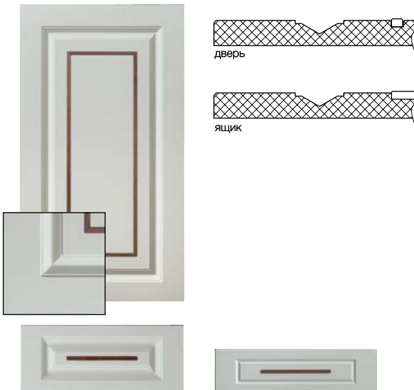
Рис. 335 Максимальный размер фасада 2750x1200
