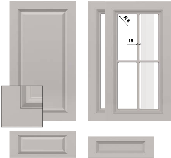
Рис. 35* Максимальный размер фасада 2750х1200
