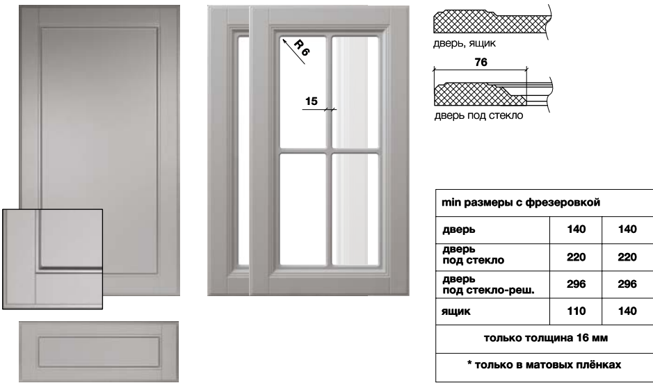
Рис. 47-1* Максимальный размер фасада 2750x1200
