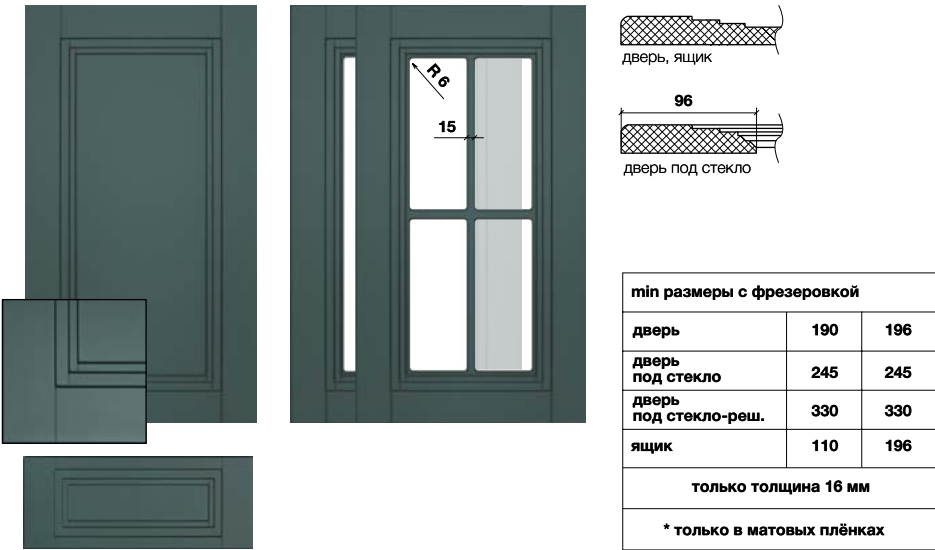
Рис. 48* Максимальный размер фасада 2750x1200
