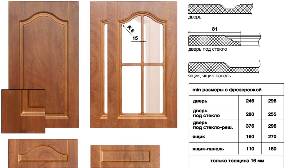
Рис. 15-3 Максимальный размер фасада 2750x1200
