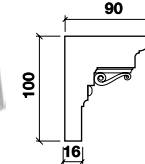
карниз 05 ДВ (100x500), R-300 (п/ш)
