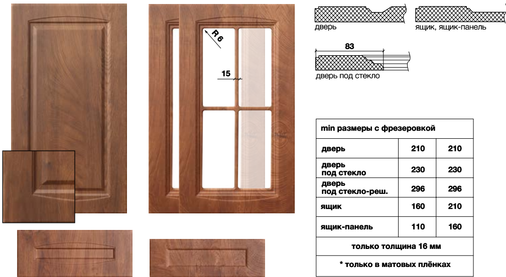
Рис. 16* Максимальный размер фасада 2750x1200
