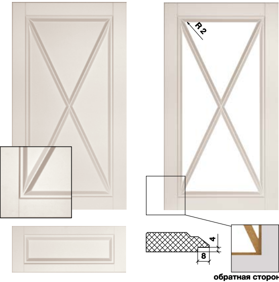
Рис. 51* Максимальный размер фасада 2750x1200
