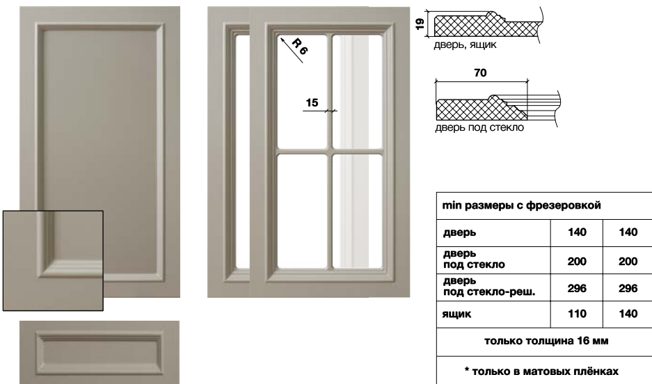
Рис. 45-3* Максимальный размер фасада 2750x1200
