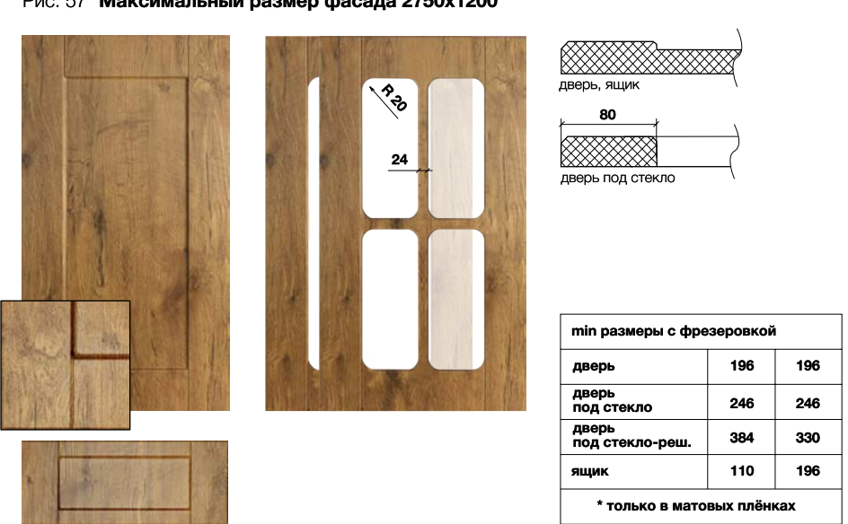
Рис. 57* Максимальный размер фасада 2750x1200
