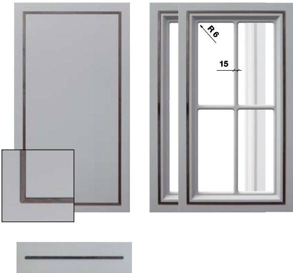
Рис. 309 Максимальный размер фасада 2750x1200
