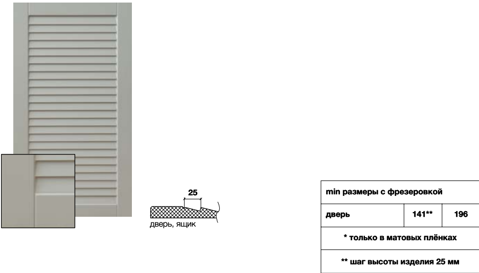
Рис. 59-1* Максимальный размер фасада 2741x1200
