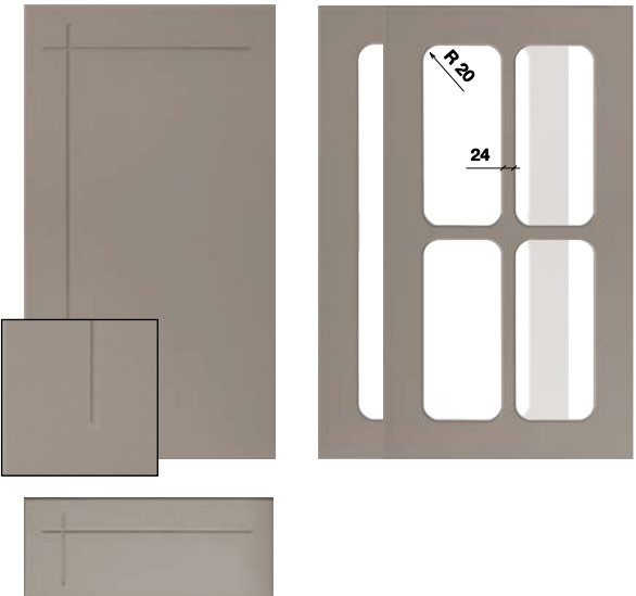
Рис. 29 Максимальный размер фасада 2750х1200
