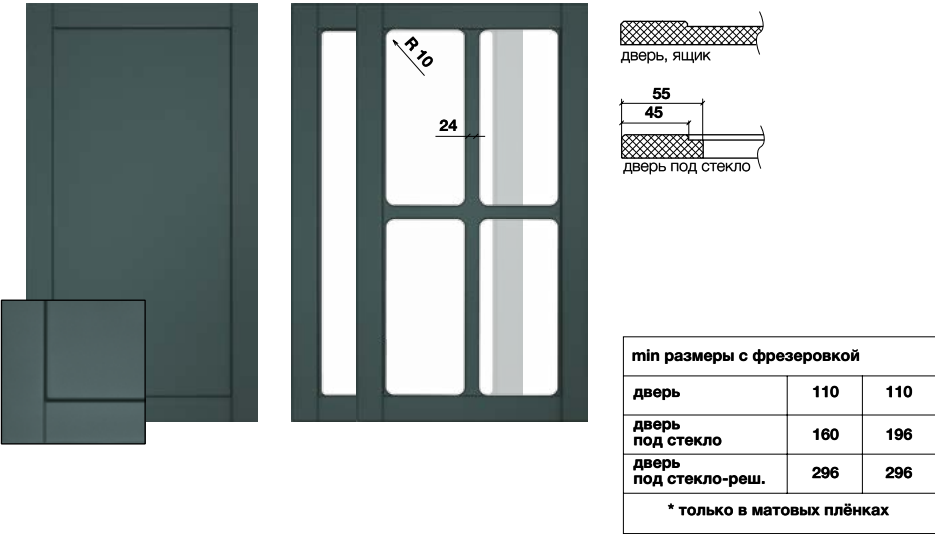
Рис. 59* Максимальный размер фасада 2750x1200
