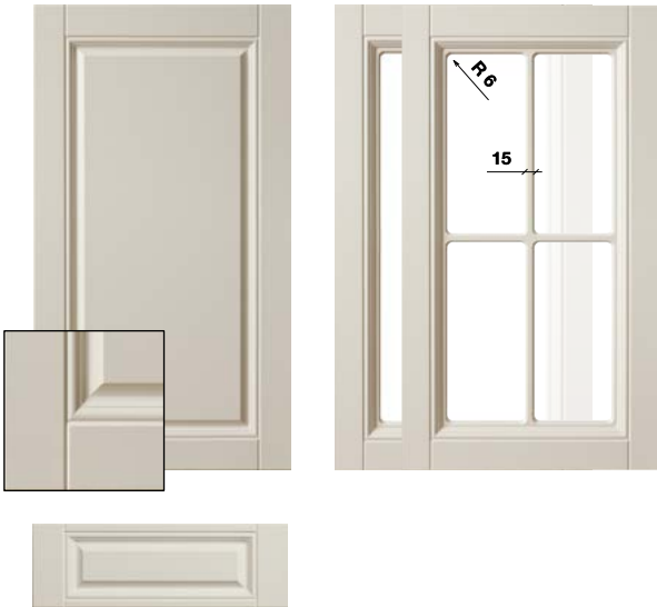
Рис. 45-5* Максимальный размер фасада 2750x1200
