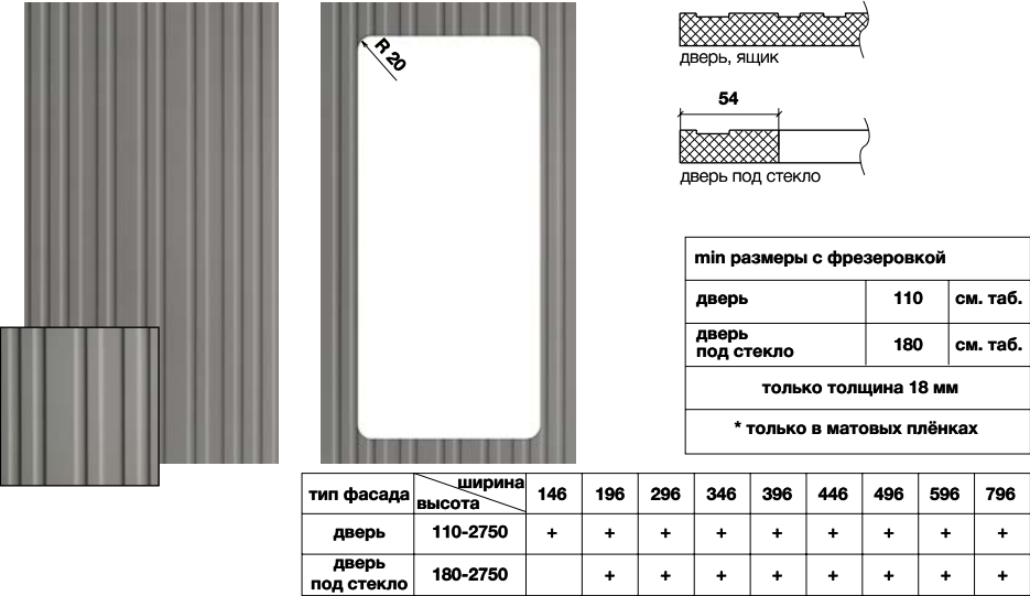
Рис. 60* Максимальный размер фасада 2750x1200
