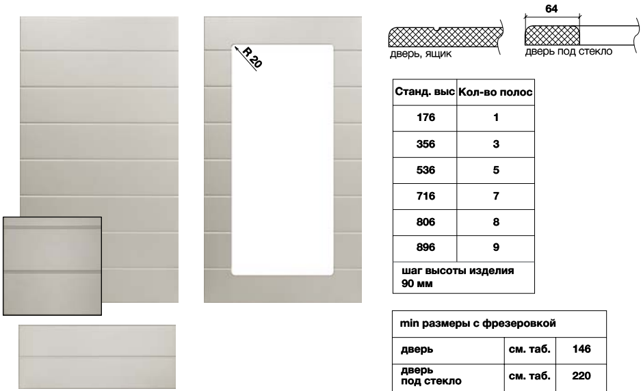
Рис. 25 Максимальный размер фасада 2750x1200
