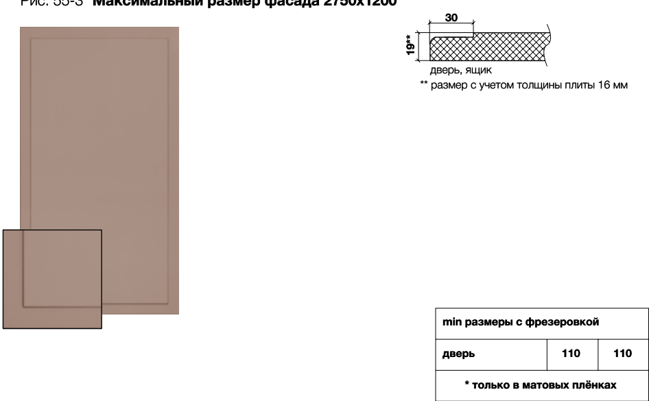
Рис. 55-3* Максимальный размер фасада 2750x1200
