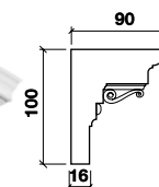
карниз 05 ДУ (100x500), R-300 (п/ш)
