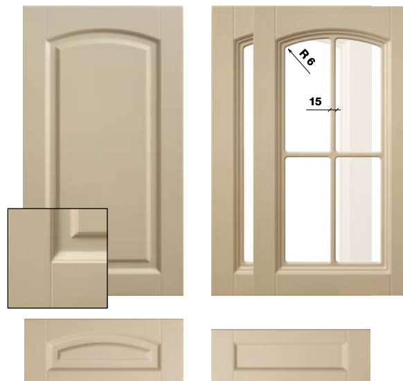
Рис. 15-2* Максимальный размер фасада 2750x1200
