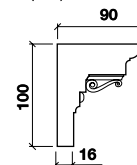
карниз 05 ДВ (100х500), R-300 (п/ш)
