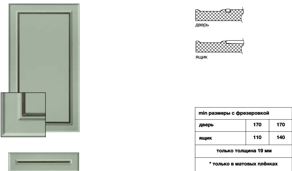
Рис. 355-1 Максимальный размер фасада 2750x1200
