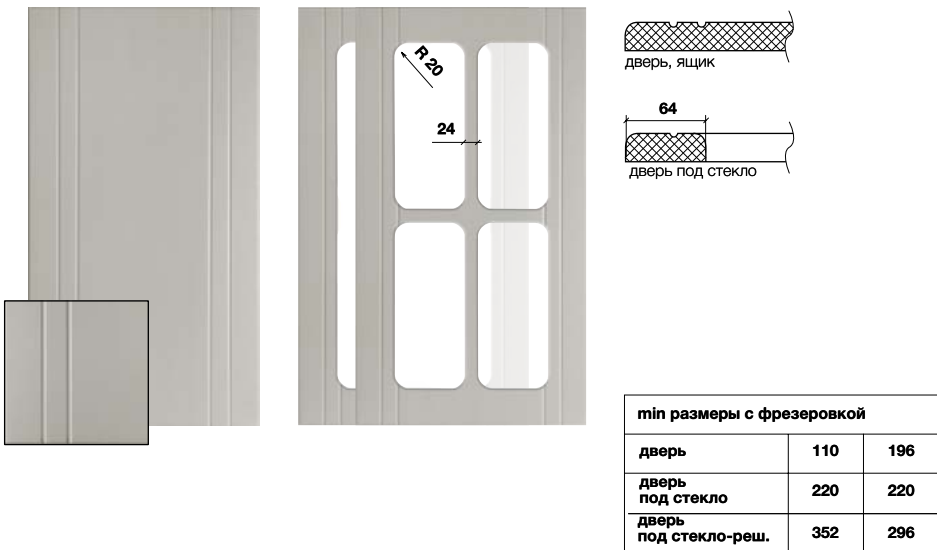
Рис. 27 Максимальный размер фасада 2750x1200
