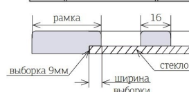
2-решетка (число окон зависит от ширины решетки)
