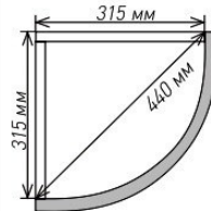
ящик верхнего ряда
